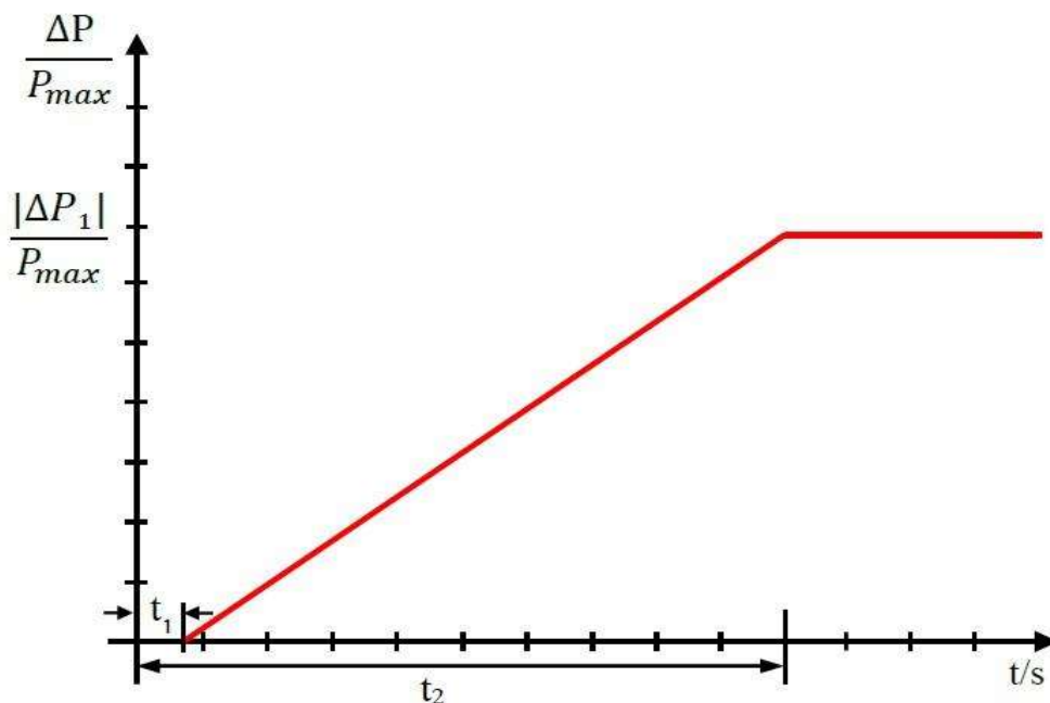
Obr. 3: Schopnost frekvenční odezvy činného výkonu u vysokonapěťové stejnosměrné soustavy. \Delta P je změna činného výkonu vyvolaná skokovou změnou frekvence.
